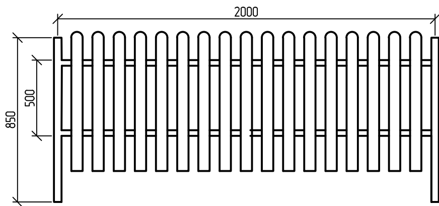
Ограждение деревянное
